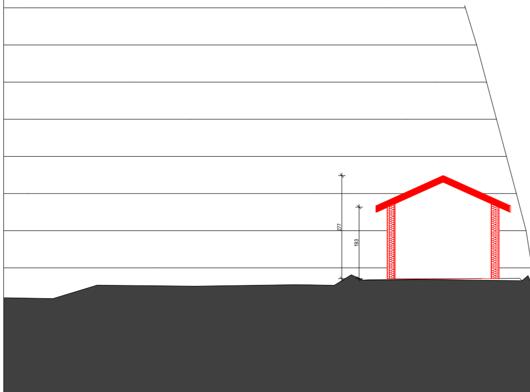
Coupe AA
